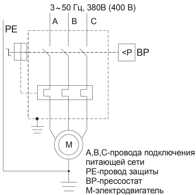
Рисунок А.1 - Схема электрическая принципиальная компрессоров СБ4/С-100.LB75, СБ4/Ф-270.LB75, СБ4/Ф-270.LB75В, СБ4/Ф-500.LB75
