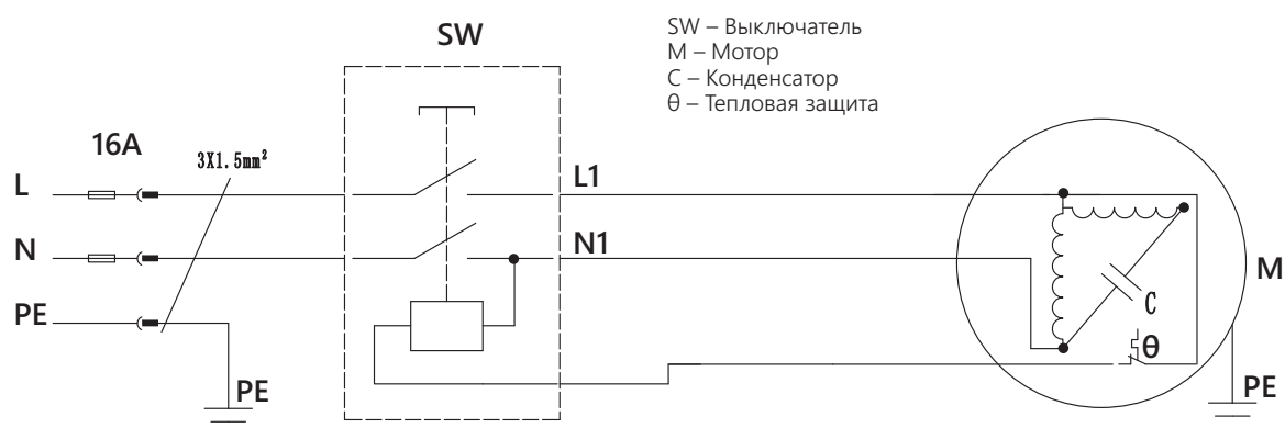
Рисунок 19. Модель BELMASH TS-250P и BELMASH TS-250PE.
