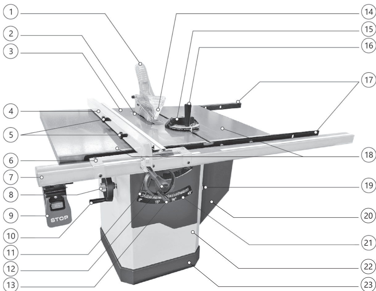
Рисунок 1. Основные элементы станка BELMASH TS-250P, BELMASH TS-250P/400.
