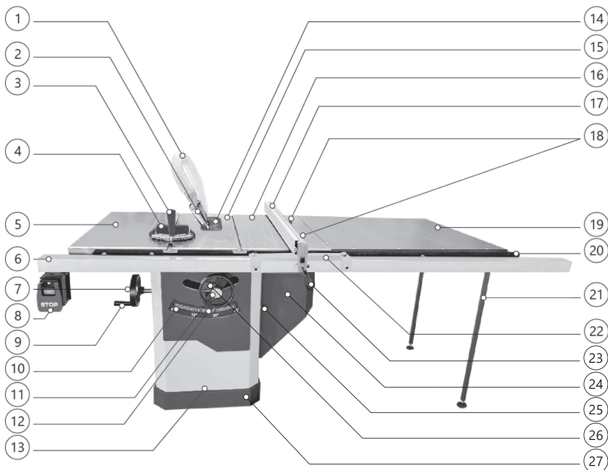
Рисунок 2. Основные элементы станка BELMASH TS-250PE, BELMASH TS-250PE/400.
