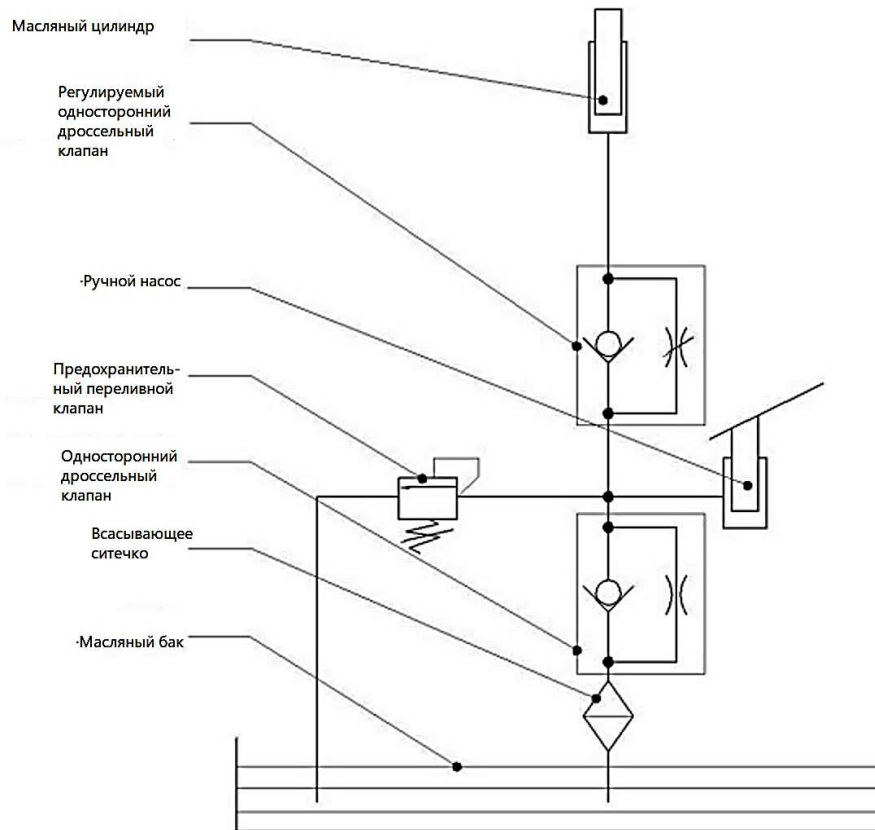
Рис.2 - Схема гидравлической системы
